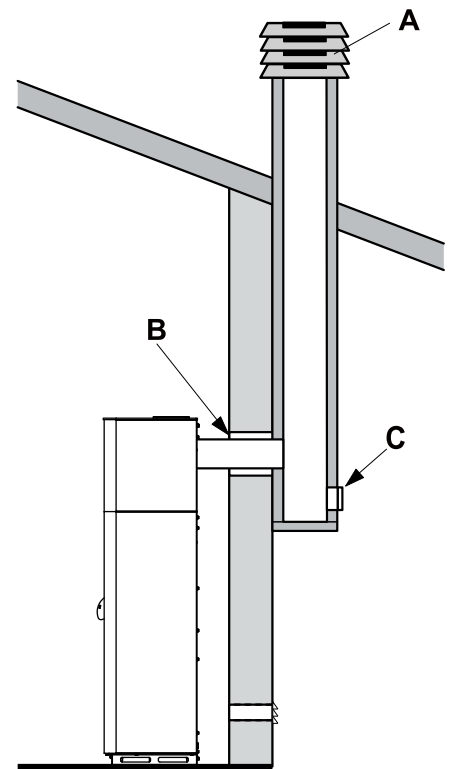
A) Windschutz-Schornsteinkopf B) Abdichten C) Inspektion fig. 5.8
