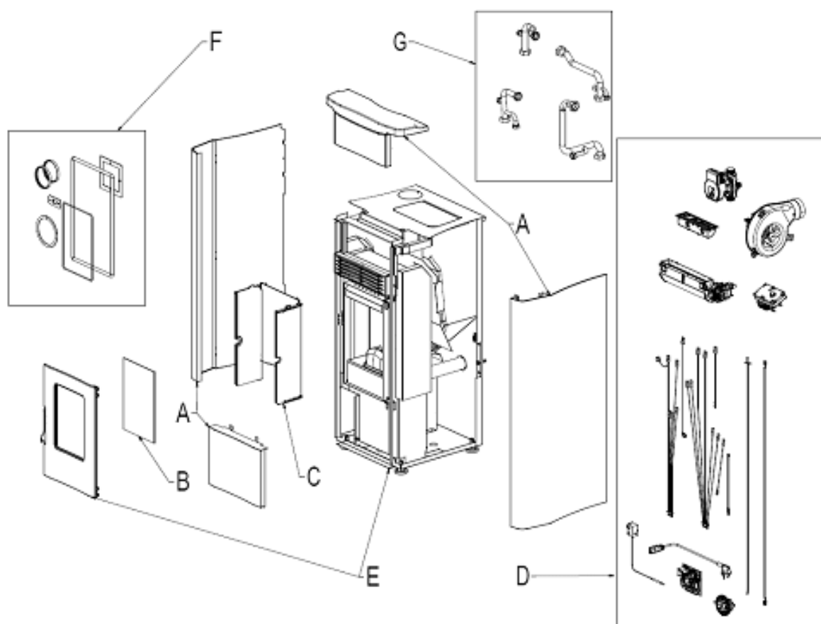
Fig. 1 - Explosionszeichnung
