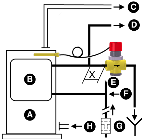
Ilustracja 1: Kocioł ze zintegrowanym grzewczakem wody pitnej
