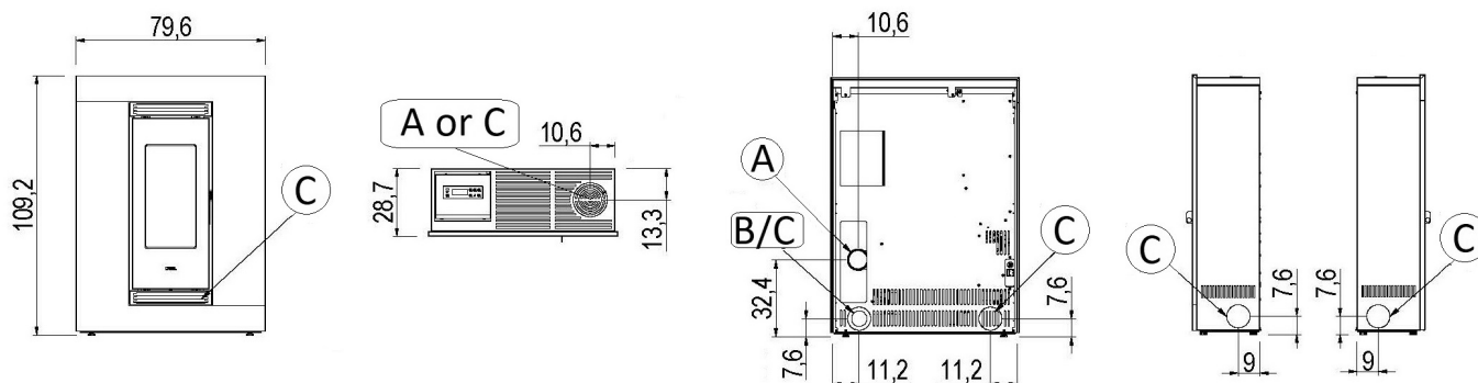
Fig. 13 - Allgemeine Abmessungen: Luce Plus 9
