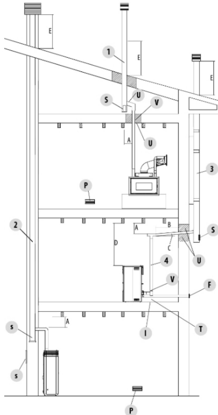
Fig. 11 - Rauchabzug
