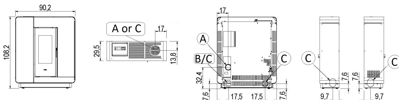
Fig. 14 - Allgemeine Abmessungen: Elle Plus 9
