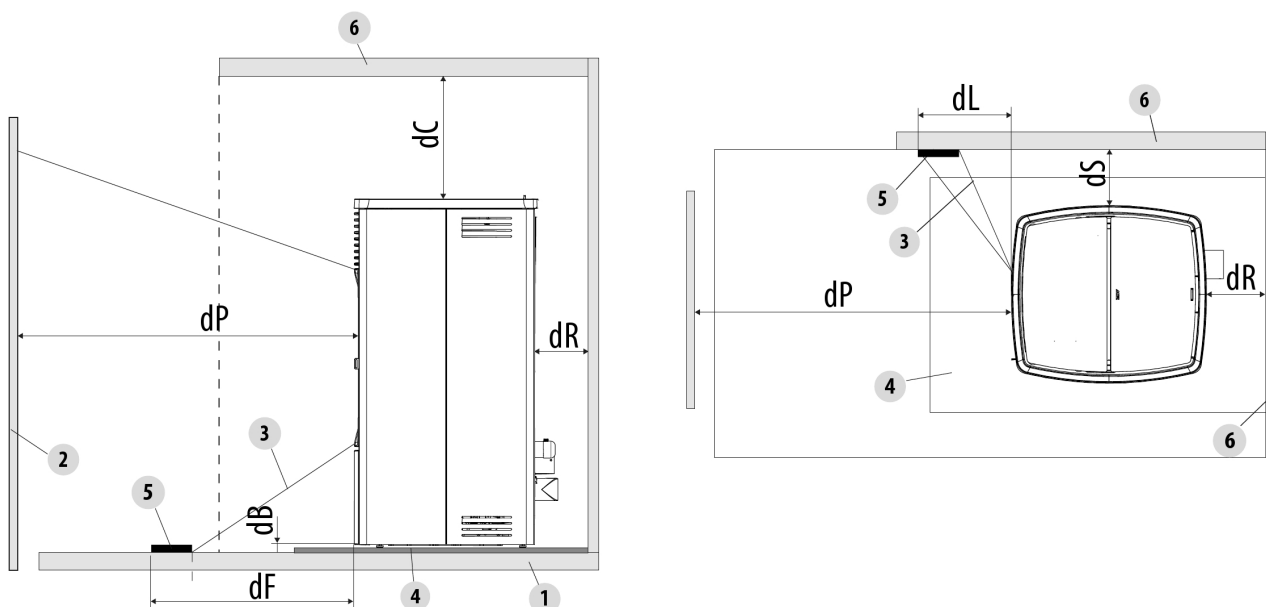
Fig. 12 - Sicherheitsabstand vom Brennstoff
