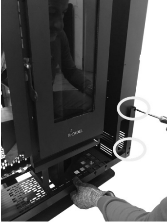
Fig. 26 - Befestigung des unteren Bügels
