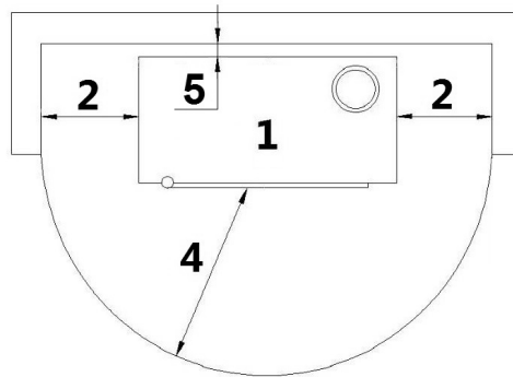
Fig. 54 - Wandinstallation
