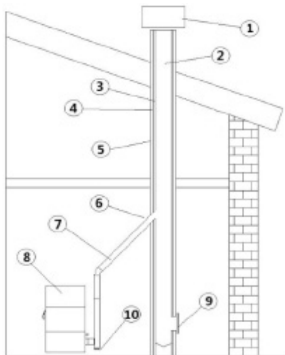
Fig. 2 - Bauteile Kamin
