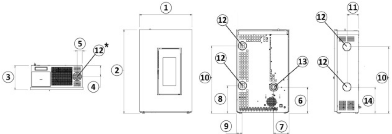
Fig. 17 - Allgemeine Abmessungen: SOLO 5 - MADISON 5
