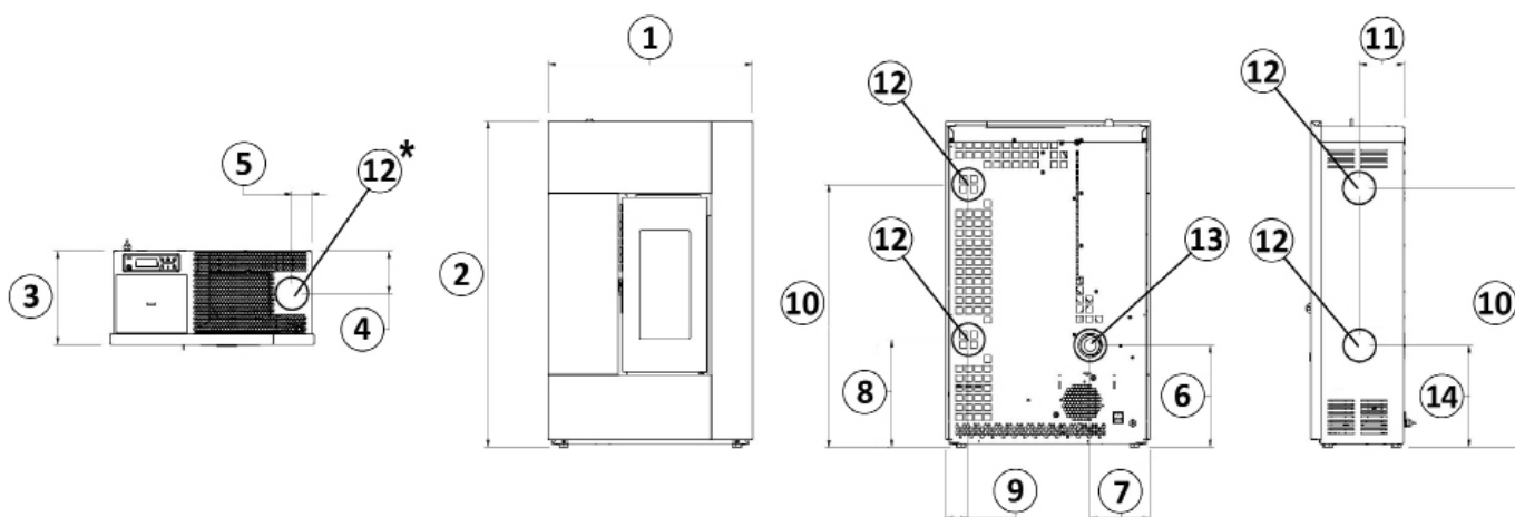
Fig. 12 - Allgemeine Abmessungen: Spirit 3
