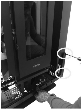
Fig. 33 - Befestigung des unteren Bügels
