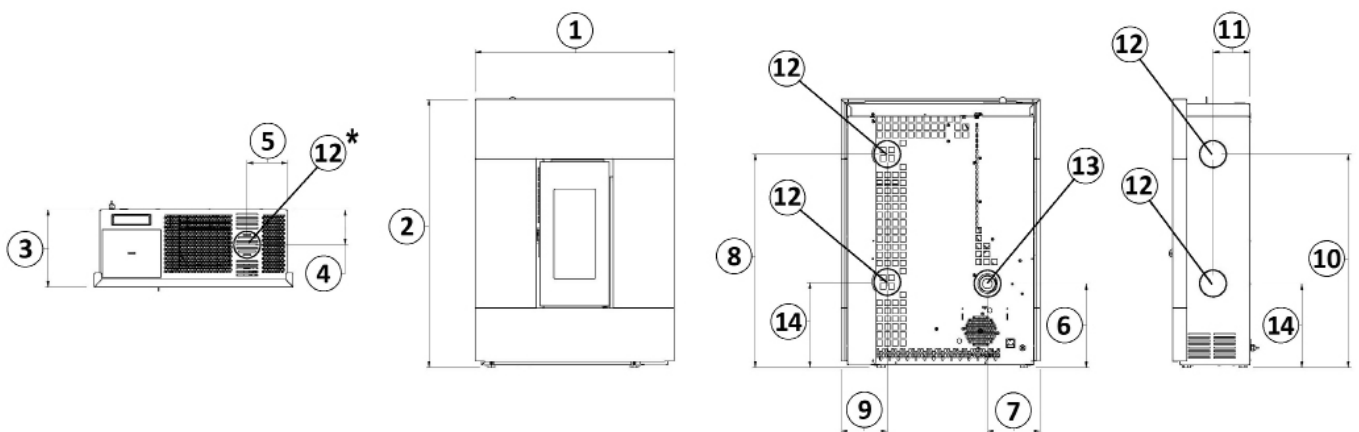
Fig. 16 - Allgemeine Abmessungen: Tabla
