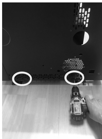
Fig. 53 - Die Schrauben befestigen
