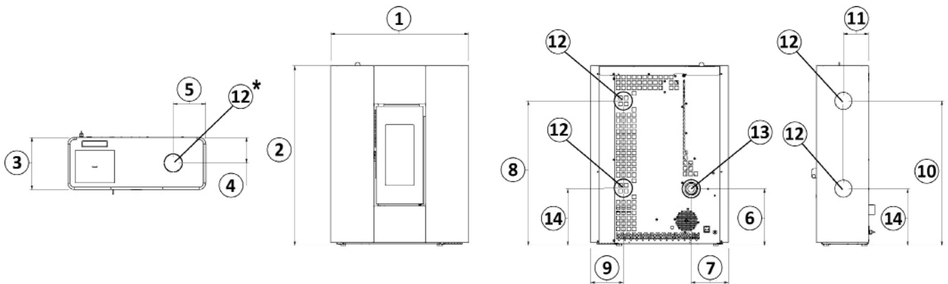
Fig. 15 - Allgemeine Abmessungen: Roxy
