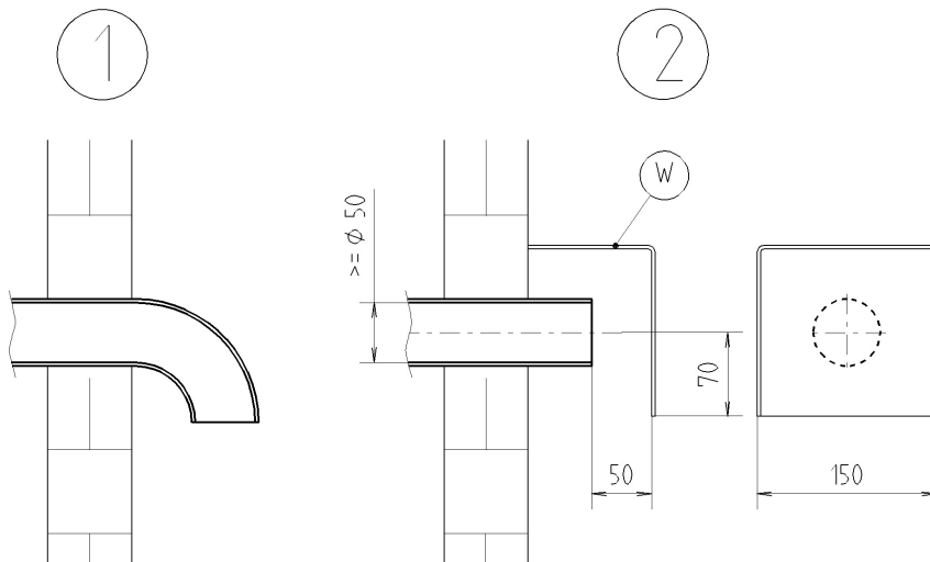
Abbildung 3: Windschutz von Zulufleitung
