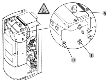
Fig. 62 - Manuelles Entlüftungsventil (unter der Abdeckplatte)
