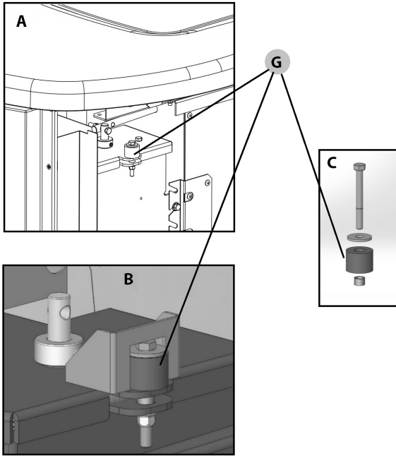
Fig. 85 - Überdruckgummi
