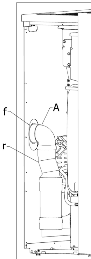
Fig. 55 - Rauchgasauslasses an der rückseite
