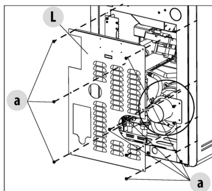
Fig. 74 - Rückwand
