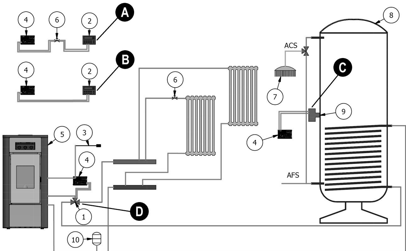
Fig. 66 - Konfiguration 2
