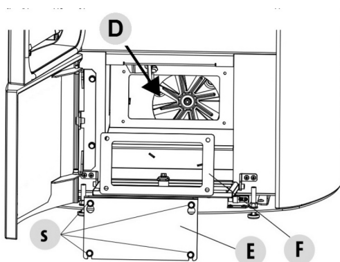
Fig. 76 - Reinigung des unteren Bereichs
