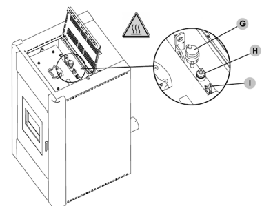
Fig. 63 - Manuelles Entlüftungsventil (unter der Abdeckplatte)
