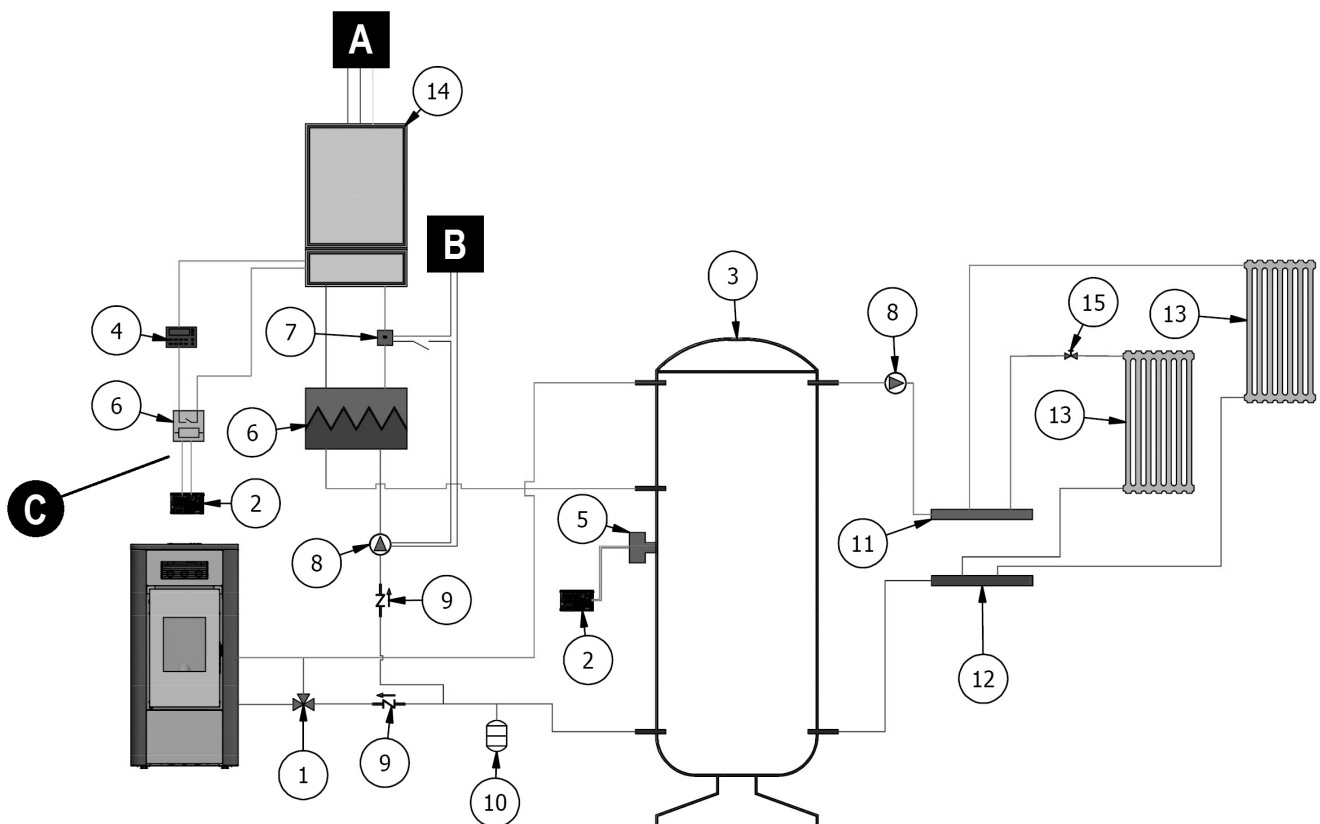
Fig. 70 - Konfiguration mit Boiler und wandmontiertem Zusatzheizkessel
