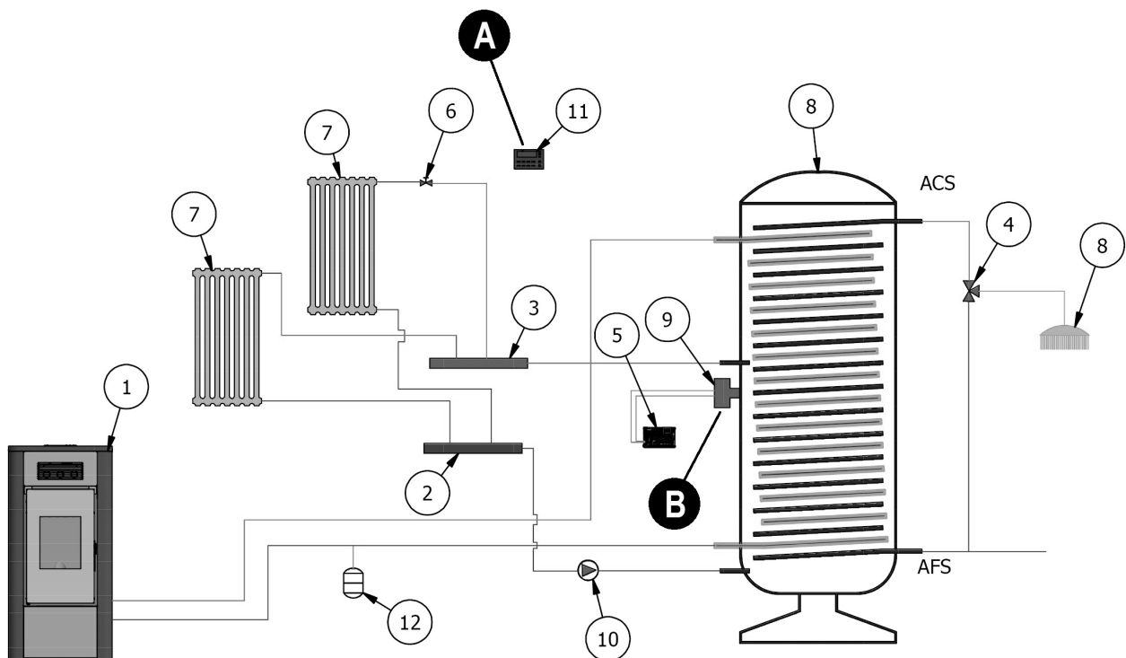
Fig. 68 - Konfiguration 4
