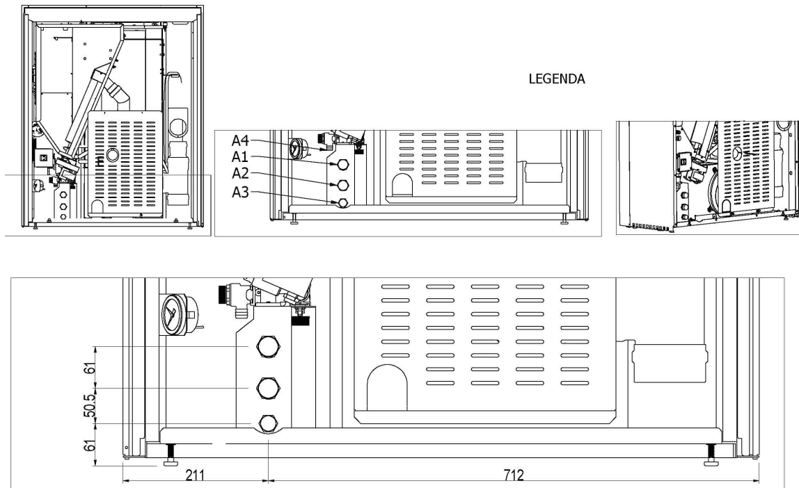
Fig. 59 - Anschlussplan
