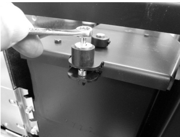
Fig. 89 - Schraube mit 8-mm-Schraubenschlüssel herausdrehen
