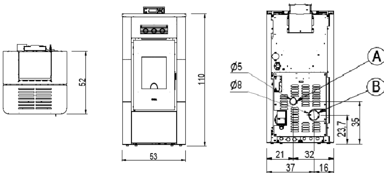
Fig. 15 - RIVER IDRO 16 - 23 - 23 H 2 O
