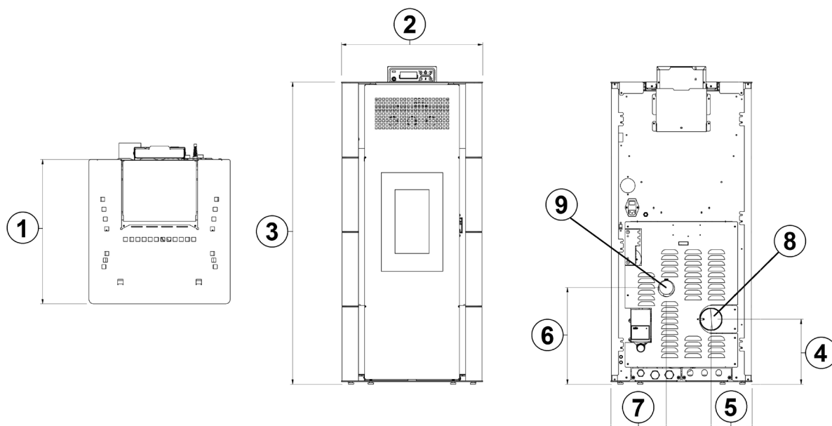
Fig. 16 - Mira 16-22 / Tesis16-23 Airtight
