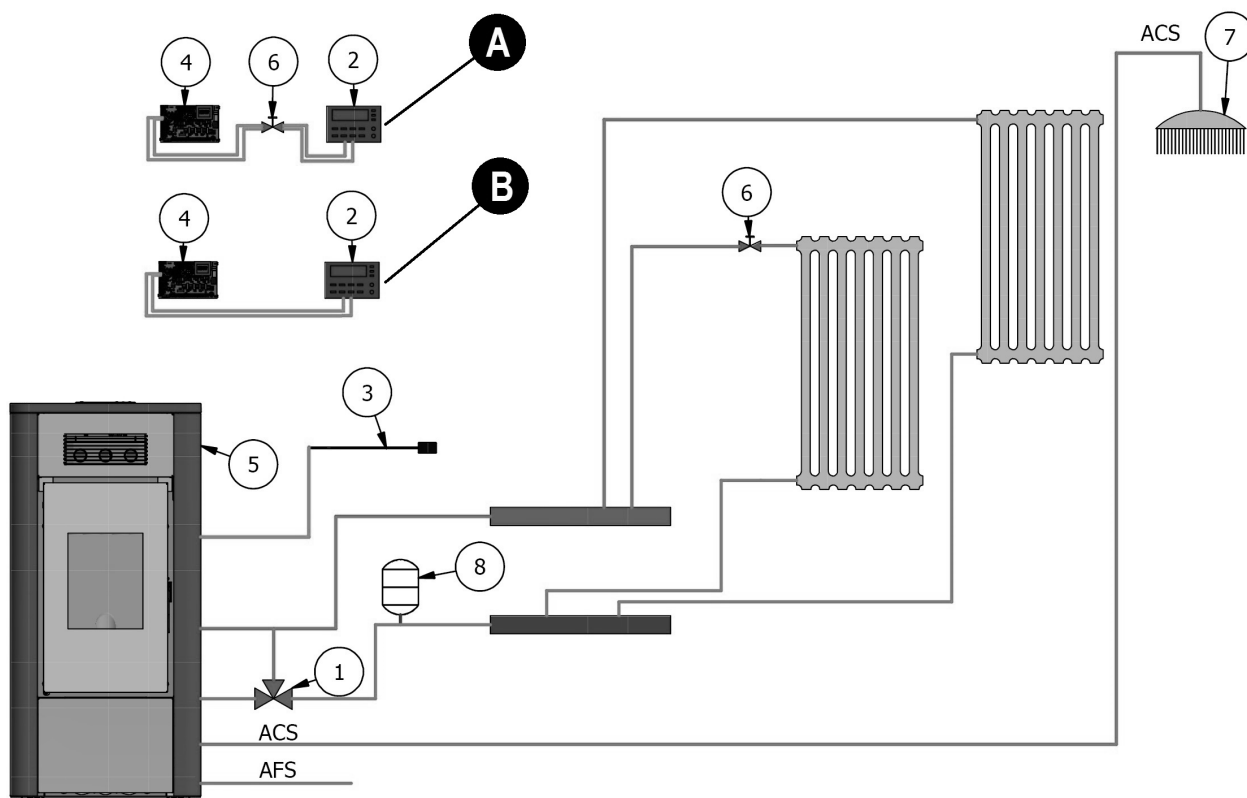
Fig. 65 - Konfiguration 2
