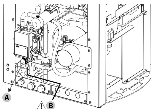
Fig. 60 - Auslassventil
