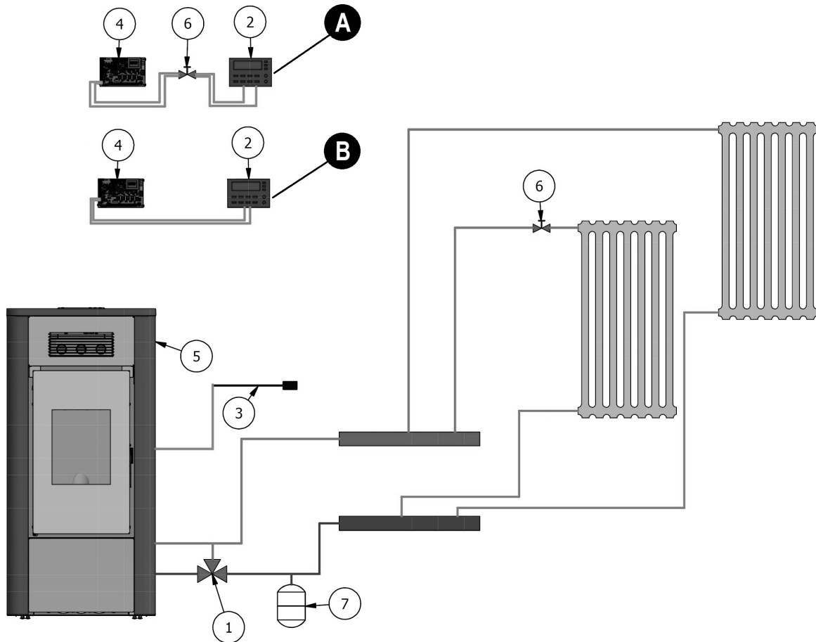
Fig. 64 - Konfiguration 1
