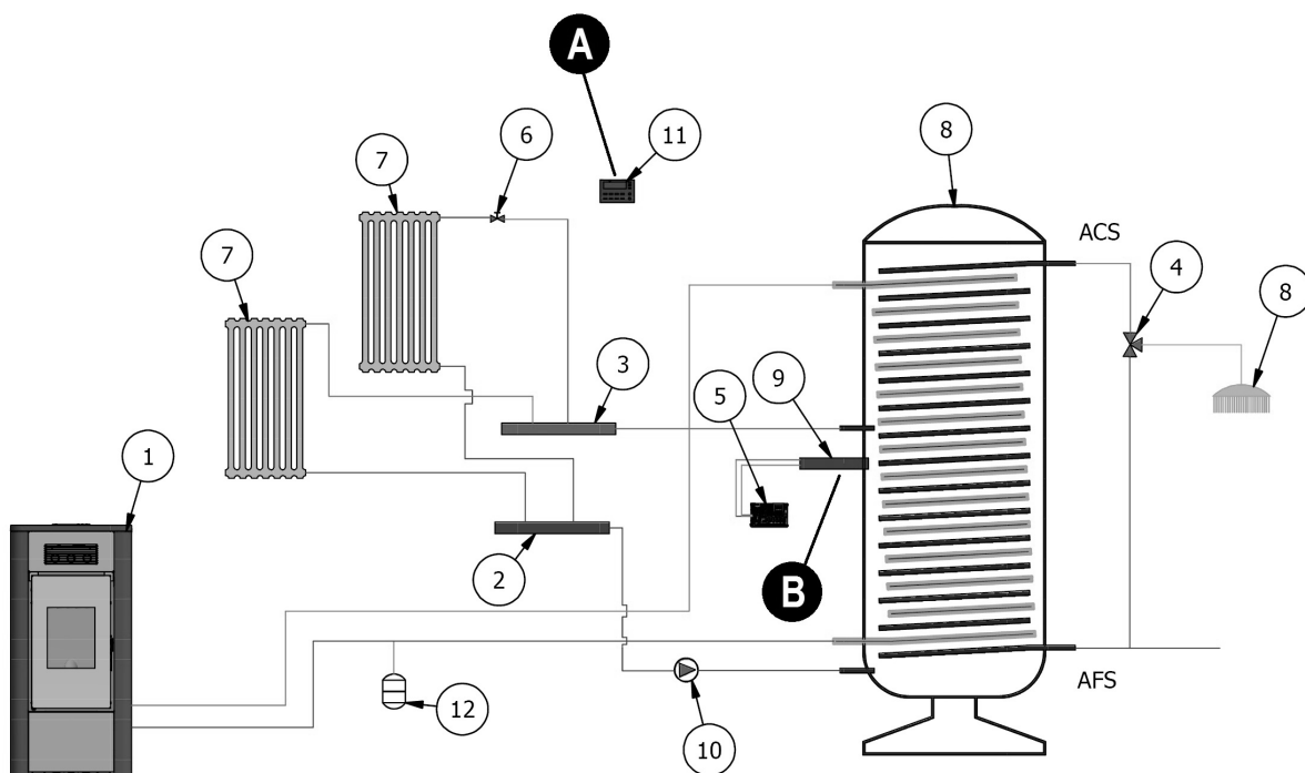
Fig. 69 - Konfiguration 5
