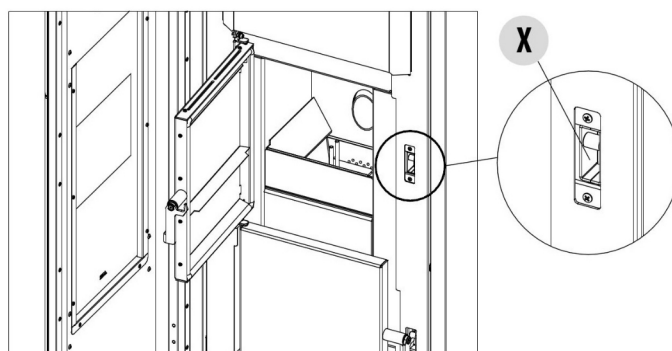
Fig. 77 - Türschließung
