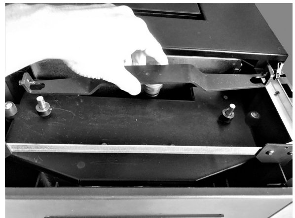
Fig. 88 - Den Griff entfernen
