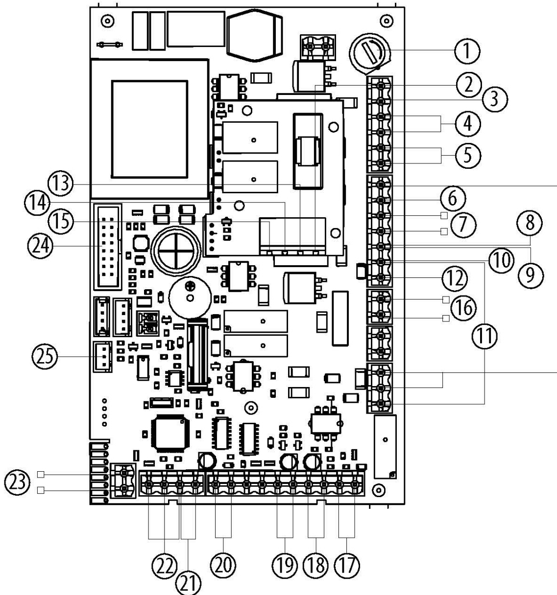
Fig. 97 - Elektrische Platine
