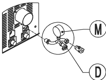
Fig. 61 - Terminal mit Ladehahn (D) und Manometer (M)
