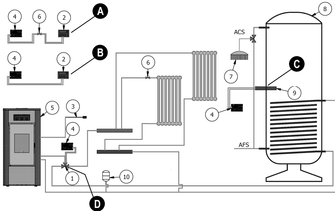
Fig. 67 - Konfiguration 3
