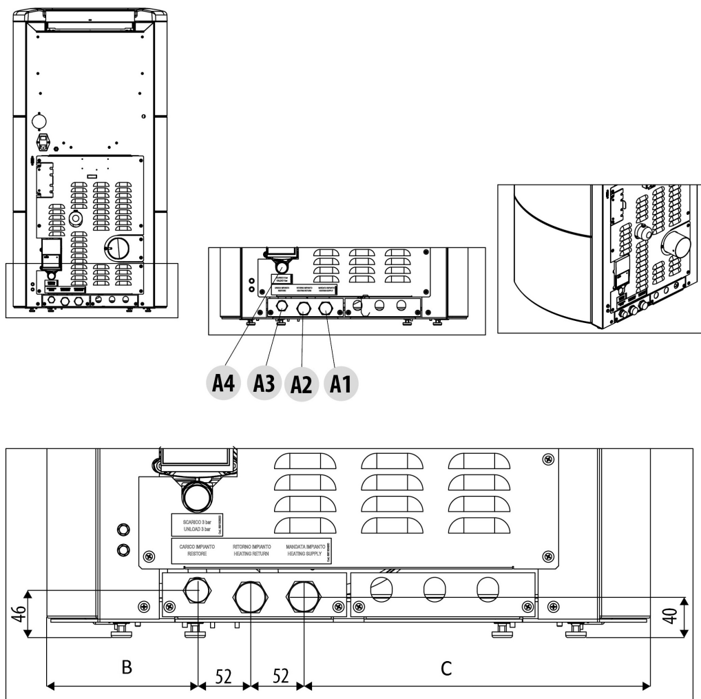
Fig. 57 - Anschlussplan
