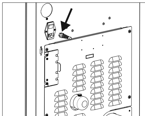
Fig. 71 - Position Sonde
