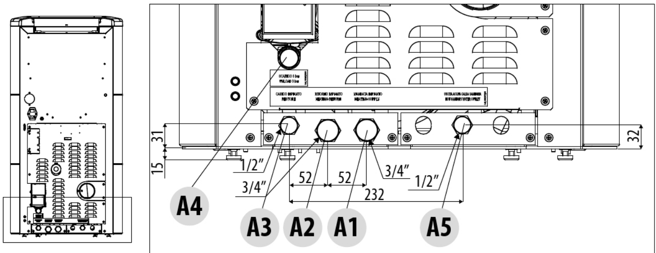
Fig. 58 - Anschlussplan mit warmwasser
