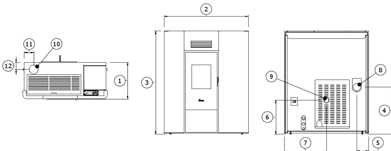
Fig. 17 - MAYA IDRO 16-24
