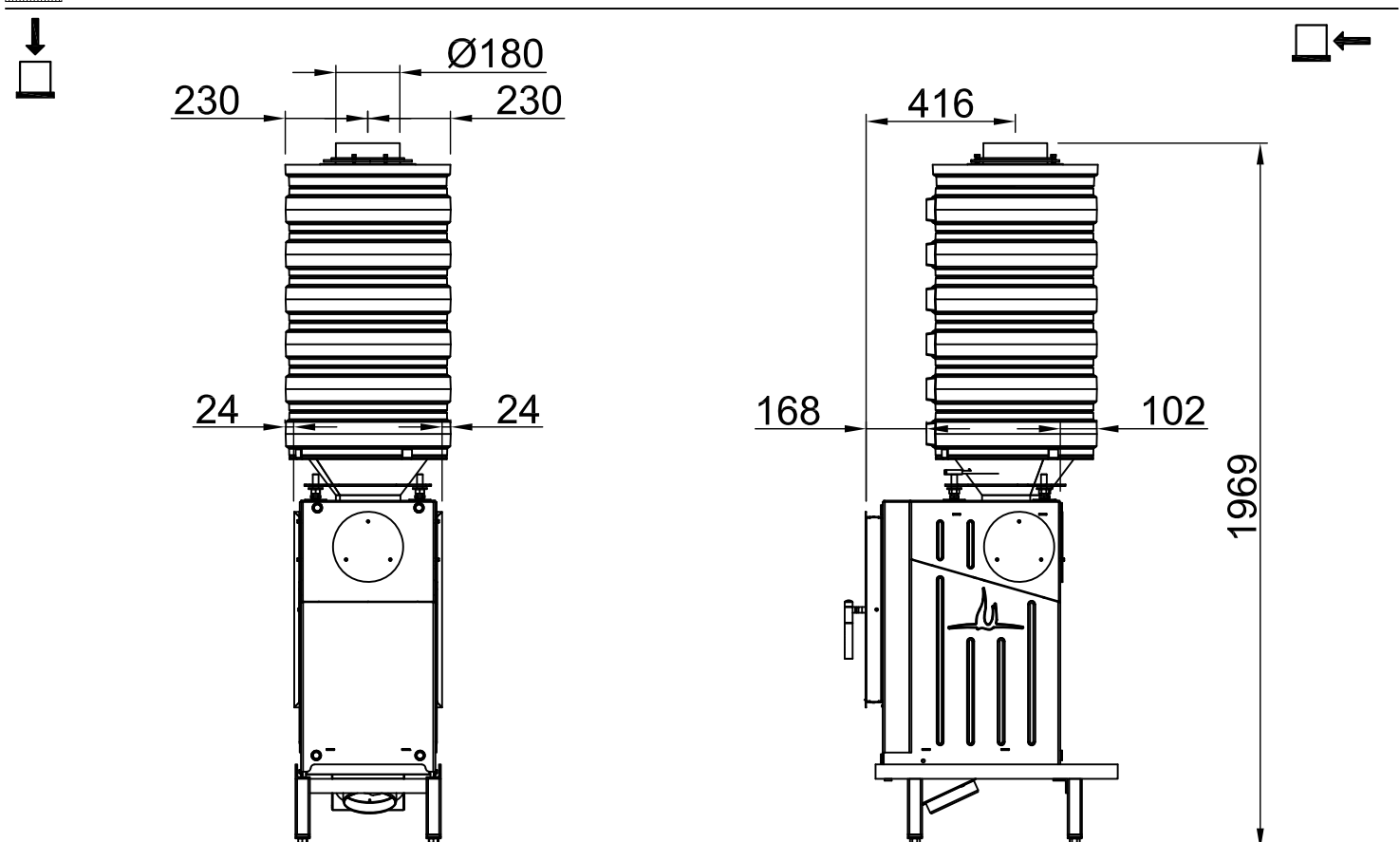
~1:20 Abgang oben, Adapter konzentrisch
