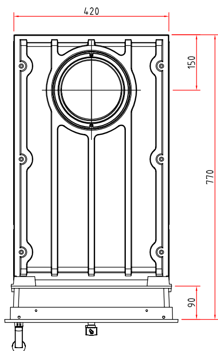
Draufsicht M 1:10
