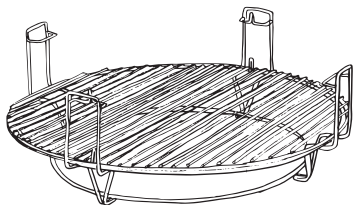
A Mit beiden halbmondförmigen Grillflächen in der unteren Ebene.
