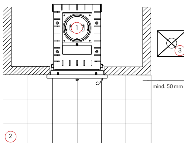
Abb.: 3 Beispiel: Schutz und Abstände vor der Feuerraumöffnung
