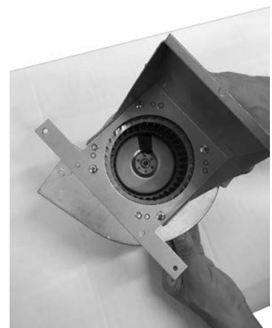
Fig. 39 - Gebläse drehen
