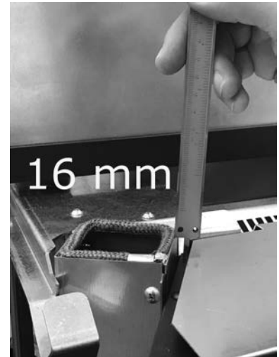
Fig. 42 - Herausragen der Luftabweichung
