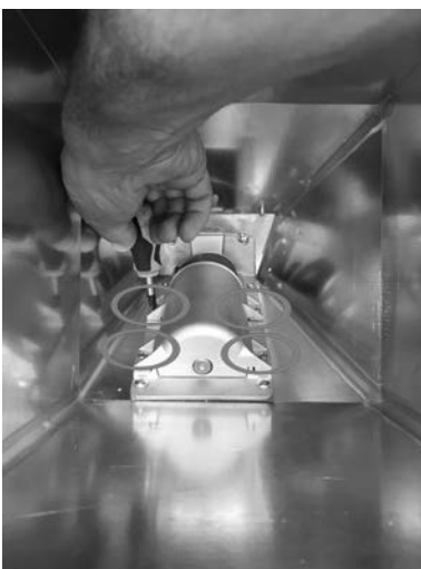
Fig. 86 - Lösen der Schrauben
