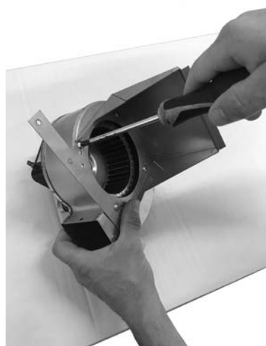
Fig. 38 - Schrauben entfernen
