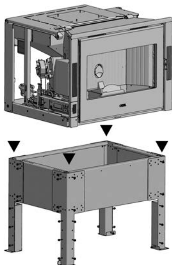
Fig. 32 - Den Einsatz oben fixieren
