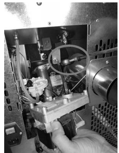
Fig. 88 - Getriebemotor entfernen
