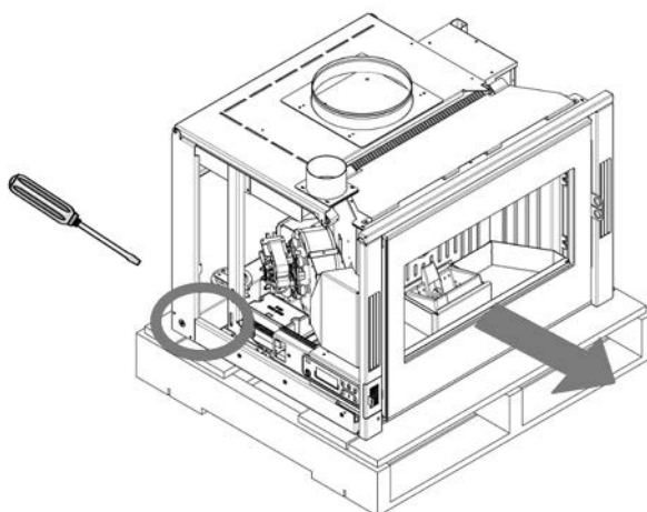
Fig. 1 - Lösen der Schrauben
