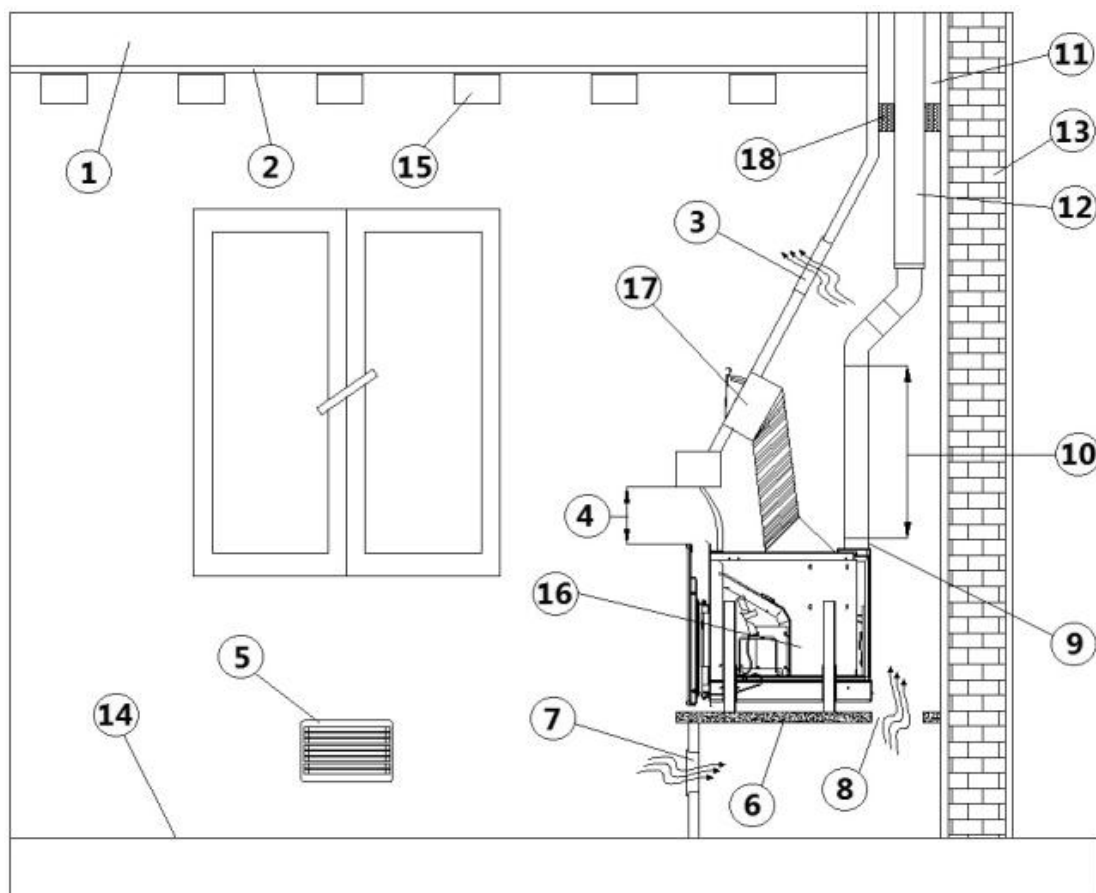
Fig. 23 - Installation an bereits vorhandenem Kamin
