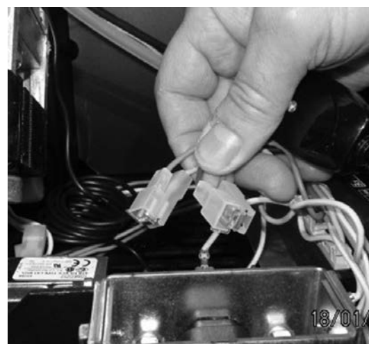
Fig. 84 - Anschluss Doppel-Faston-Buchsen
