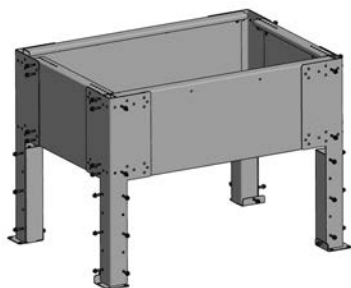
Fig. 30 - Beine zusammensetzen
