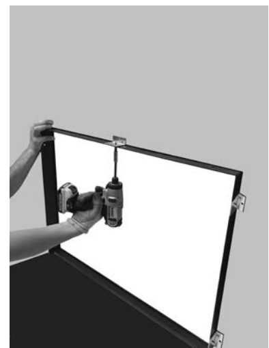
Fig. 72 - Hintere Befestigung 2
