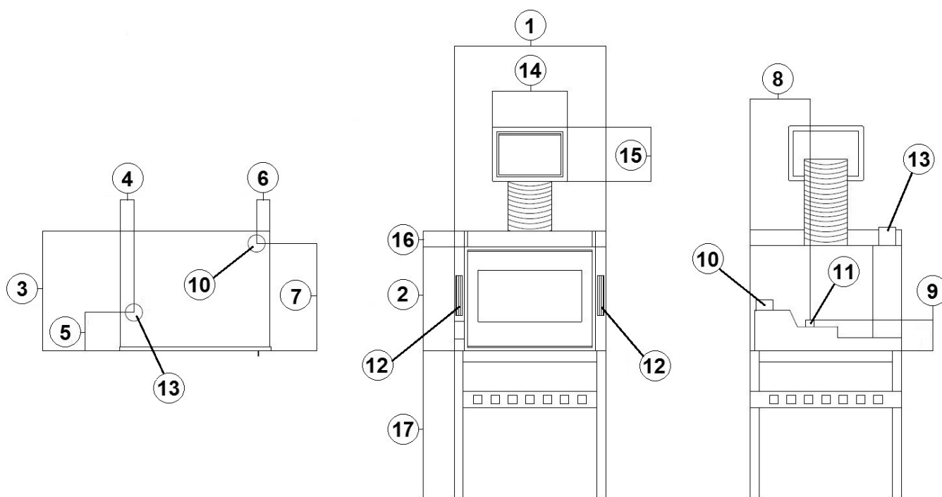
Fig. 14 - Allgemeine Abmessungen: Zefiro 3 , Zen Airtight
