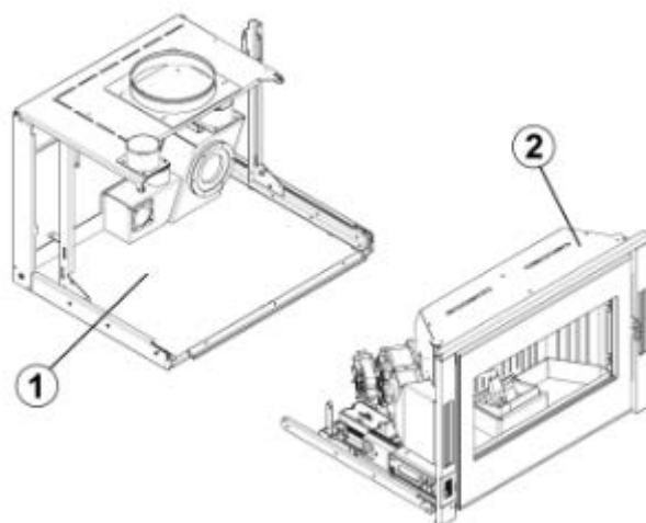
Fig. 15 - Struktur + Maschinenkörper
