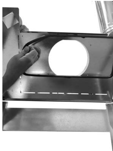
Fig. 48 - Dichtung entfernen
