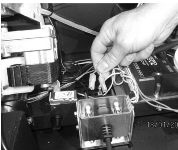
Fig. 83 - Trennen Faston-Stecker (blau - braun)
