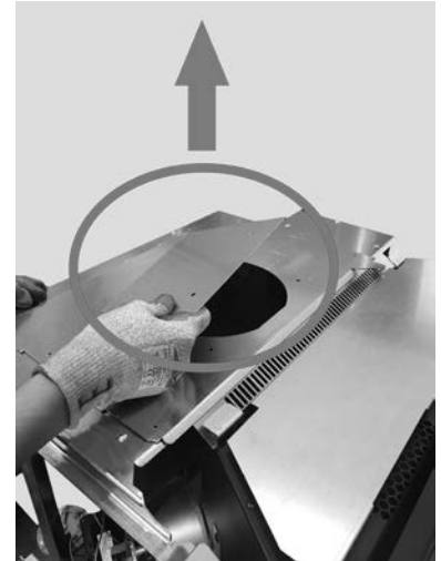
Fig. 60 - Stopfen entfernen
