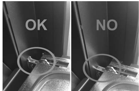
Fig. 67 - Korrektes Ankuppeln des Scharniers
