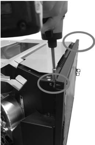
Fig. 47 - Oberes Profil entfernen
