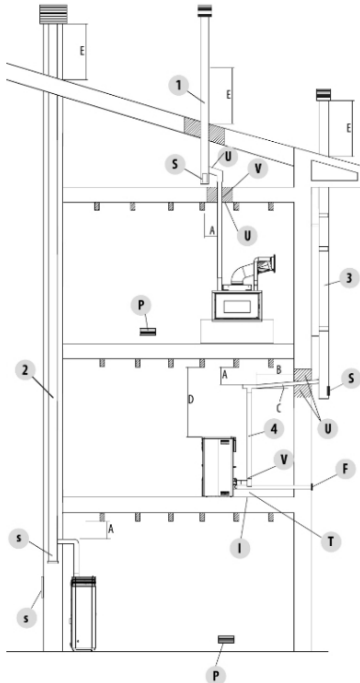
Fig. 12 - Rauchabzug
