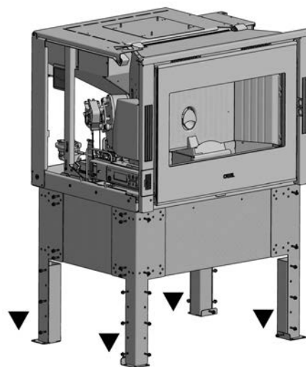
Fig. 33 - Die Struktur am Boden und an der Wand fixieren
