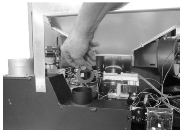
Fig. 29 - Entfernung des Rings 2
